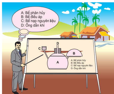
Hình 34.4. Sơ đồ hệ thống biôga xử lý chất thải trong chăn nuôi
