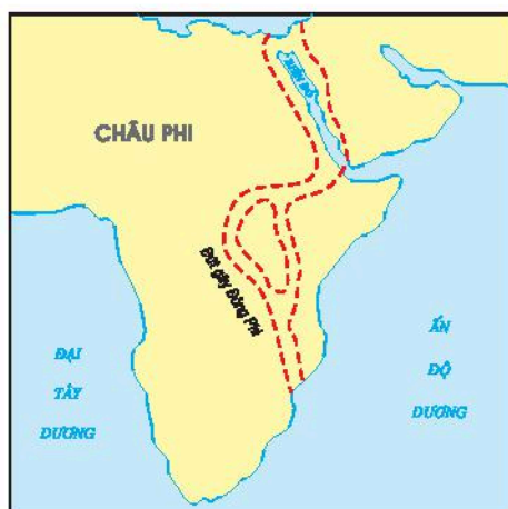
Hình 8.4 – Đứt gãy Đông Phi và Biển Đỏ
