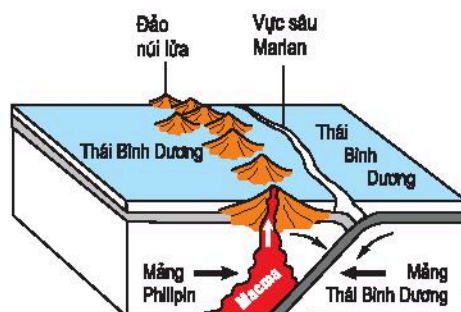
Hình 7.5 – Hai mảng kiến tạo xô vào nhau.
