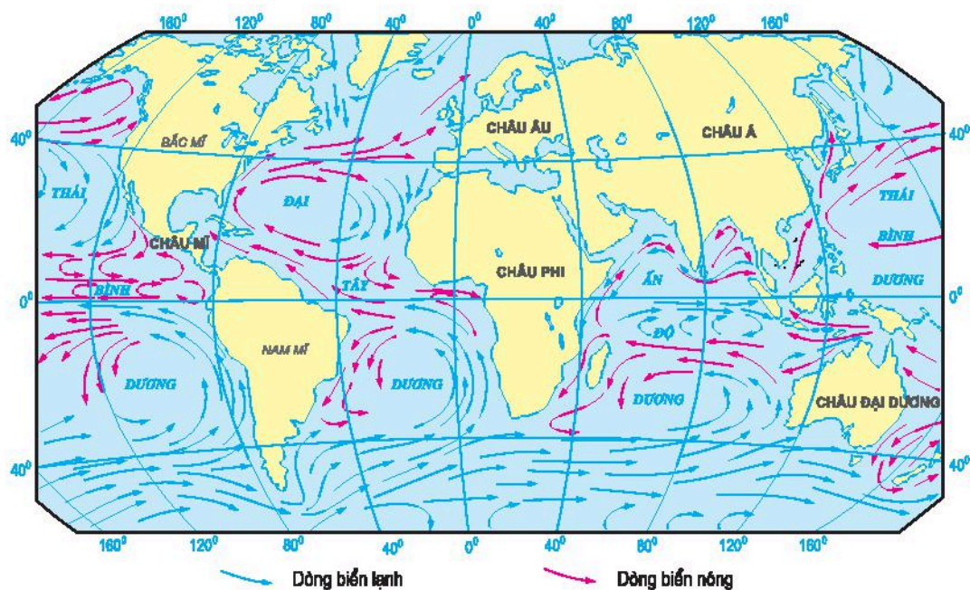
Hình 16.4 – Các dòng biển trên thế giới
