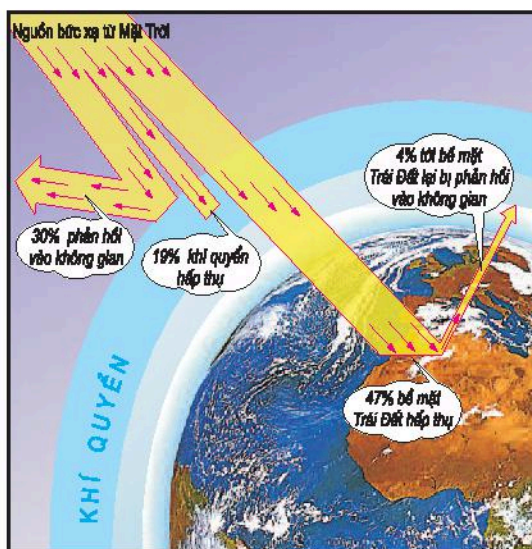
Hình 11.2 – Phân phối bức xạ mặt trời
