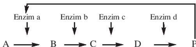
Hình 14.2. Sơ đồ minh họa sự điều hoà quá trình chuyển hoá bằng ức chế ngược.
