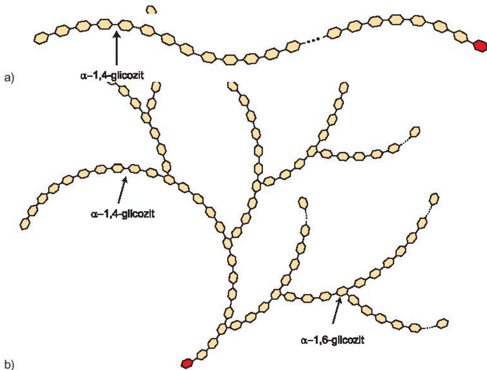
Hình 2.4. a) Mô hình phân tử amilozơ ; b) Mô hình phân tử amilopectin
