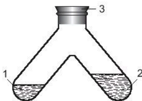
Hình 8.8. Ống nghiệm 2 nhánh dụng nước vôi trong để nhận biết \text{CO}_2 1 – Dung dịch \text{CO}_3^{2-} ; 2 – Nước vôi trong ; 3 – Nút cao su.
